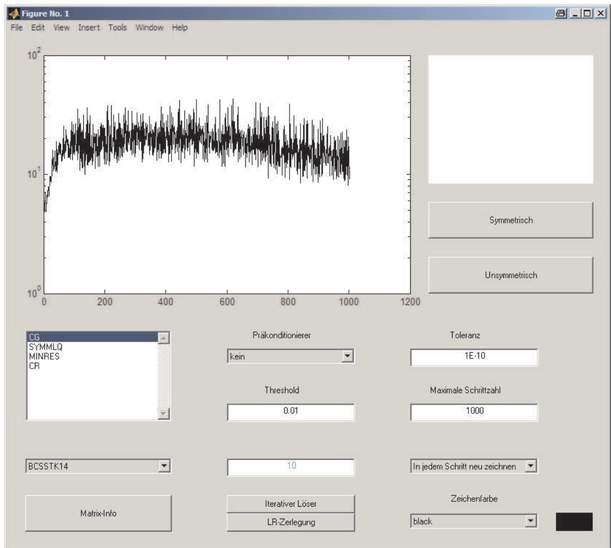
Abbildung 1: Die Programmoberfläche
